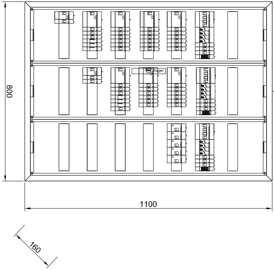
Rozdzielnica FwB IP44 II klasa
